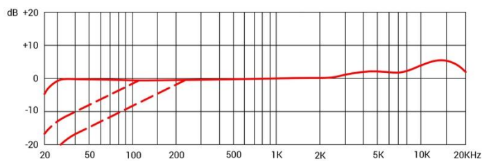
频率响应
