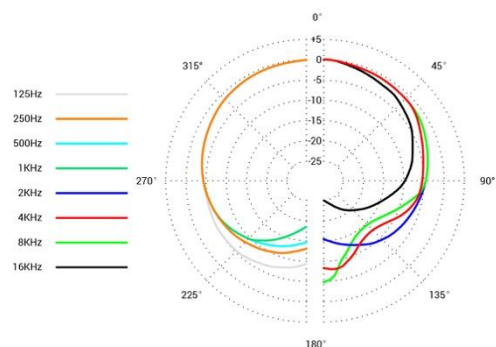
Диаграмма направленности
