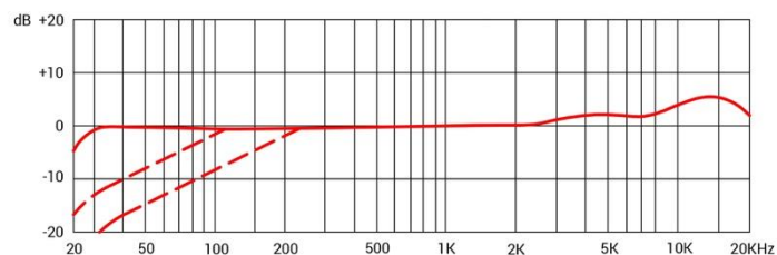
Частотный диапазон
